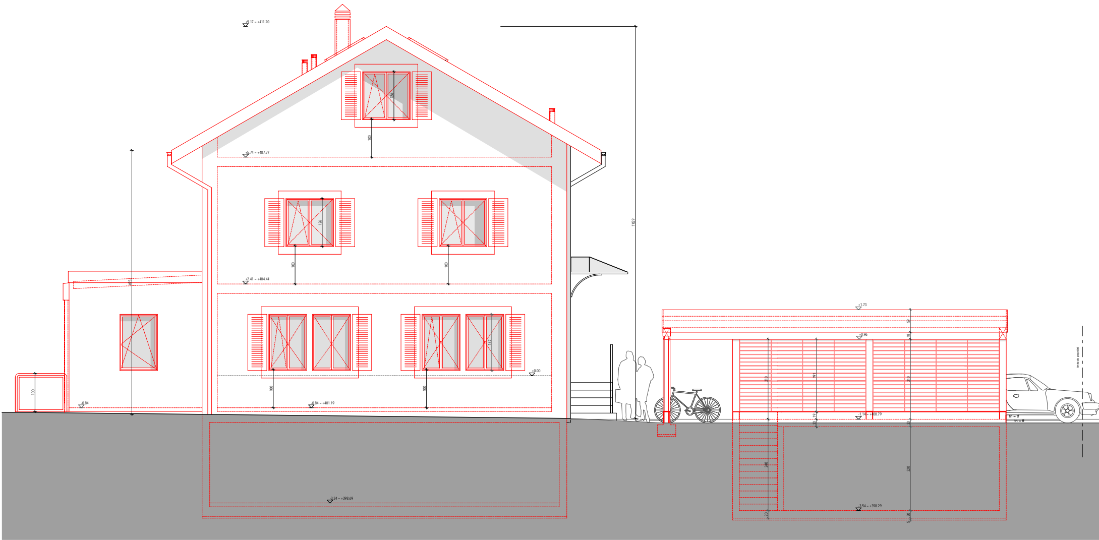
Façade nord-ouest
